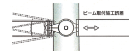
立面方向上下30° (スタンダードタイプ)
