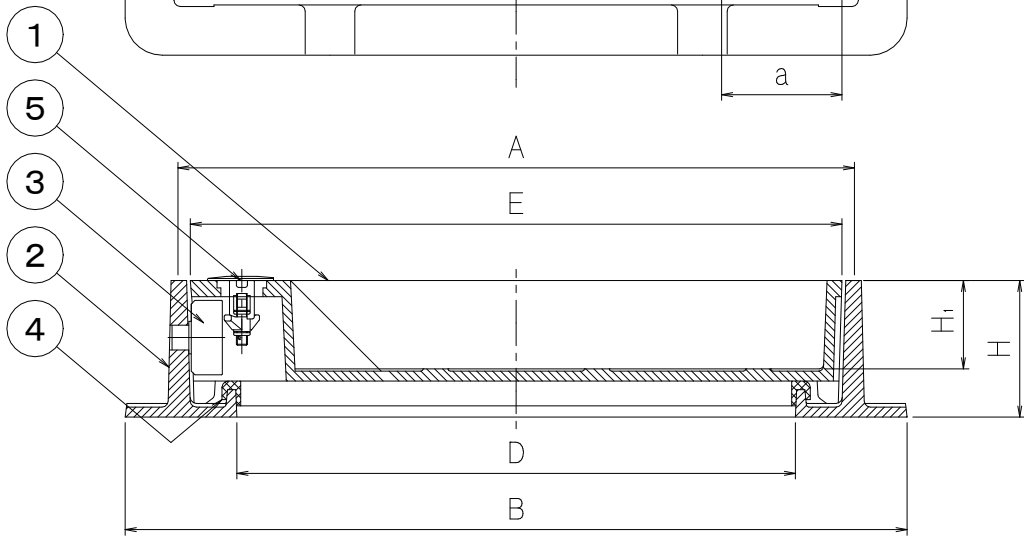
●寸法表
