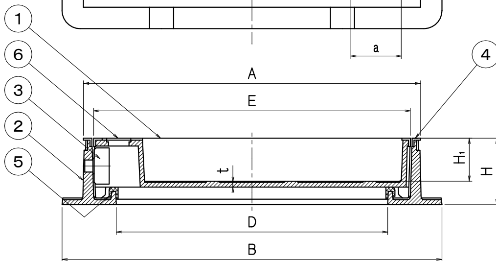
寸法表
