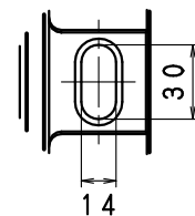
アンカー穴詳細図
