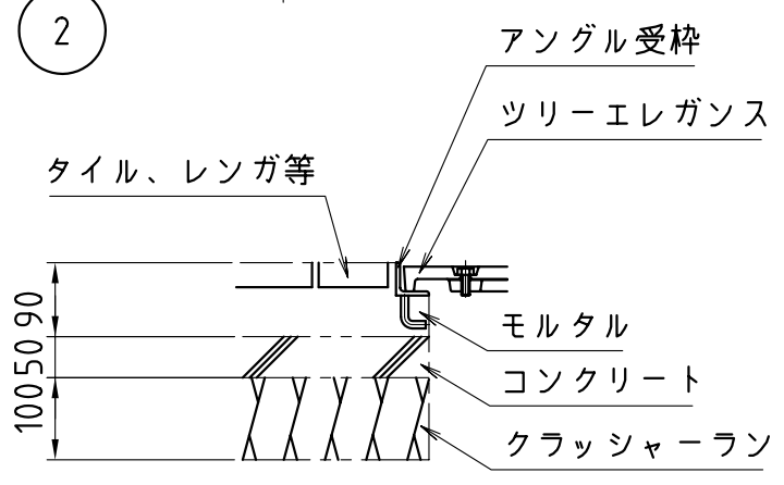
施工参考例
