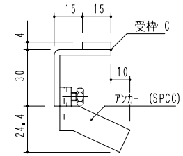
断面詳細
