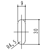
標準穴詳細
