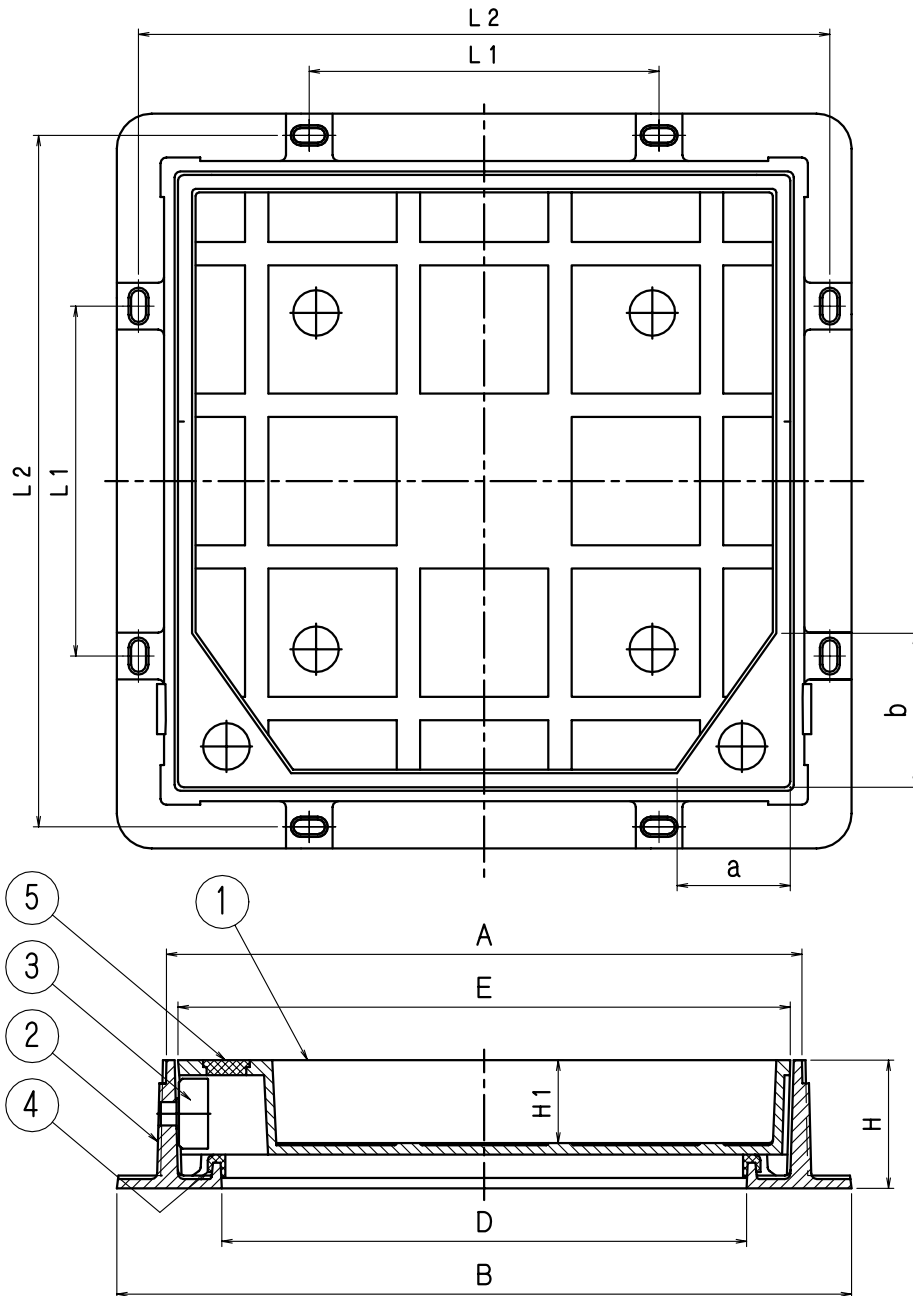
寸法表
