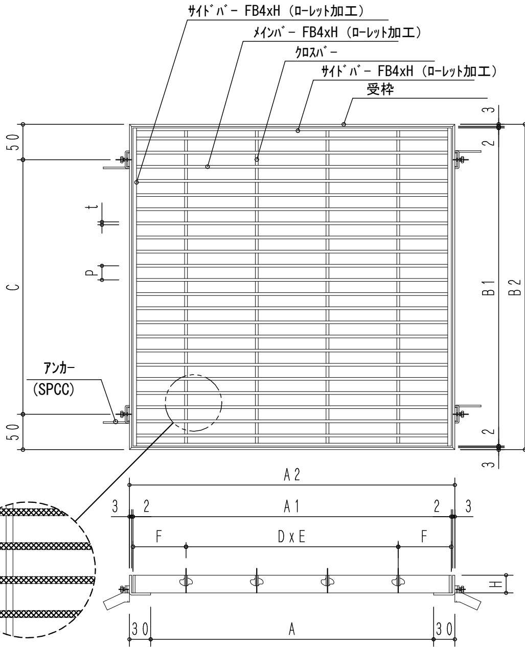
ローレット加工部拡大図
