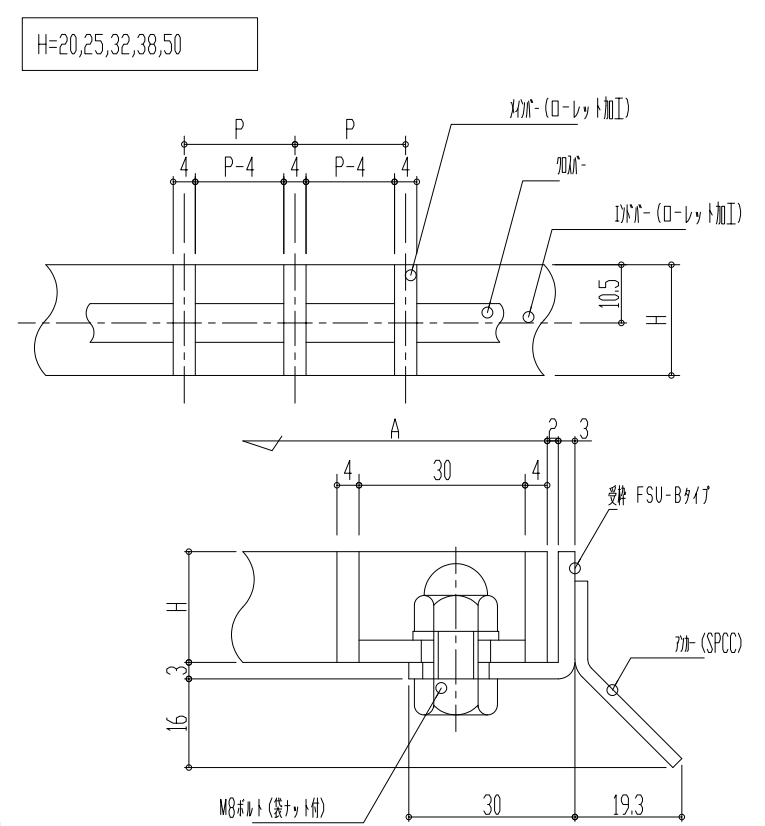
断面詳細
