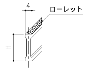
メインバ - 詳細図
