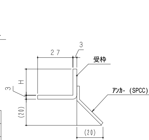
枠断面詳細図
