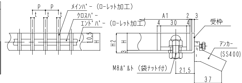
断面詳細
