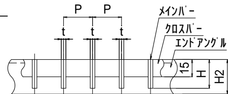
断面詳細
