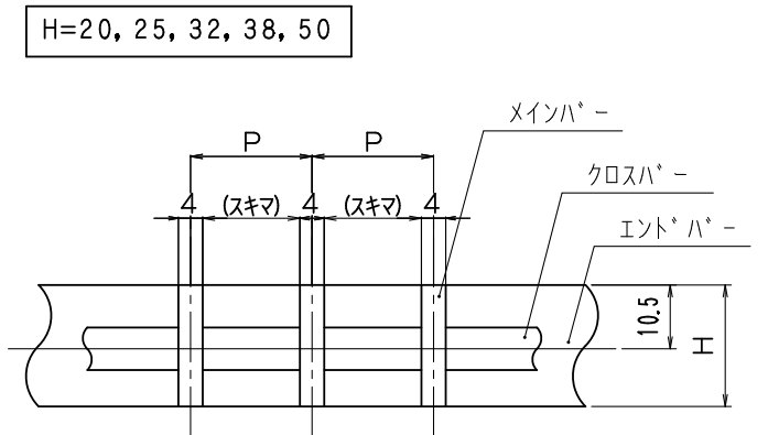
断面詳細
