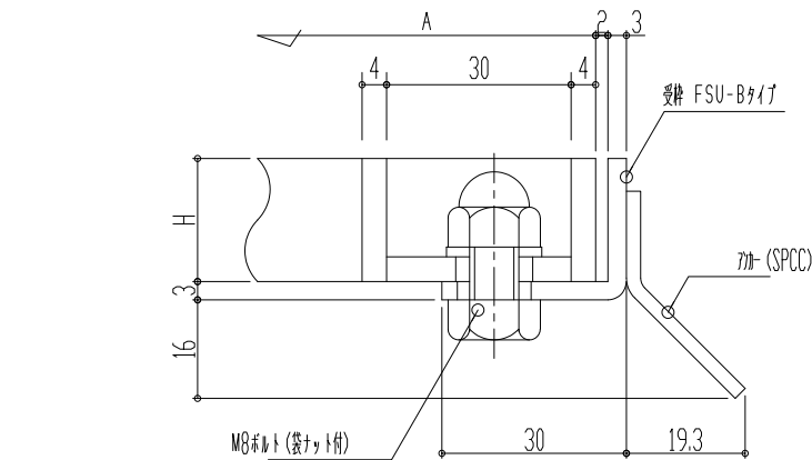
断面詳細
