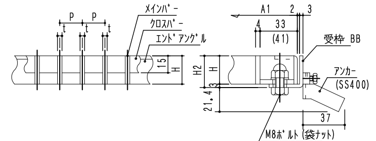
断面詳細
