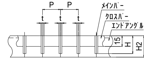
断面詳細
