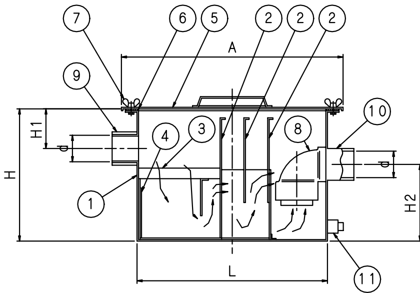
寸法表
