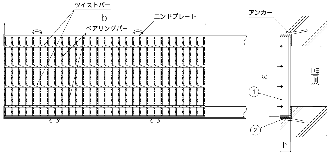
AGN横断溝用 受枠AGF
