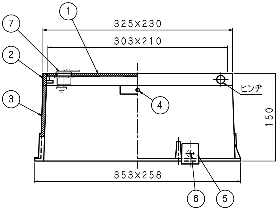
部品表
