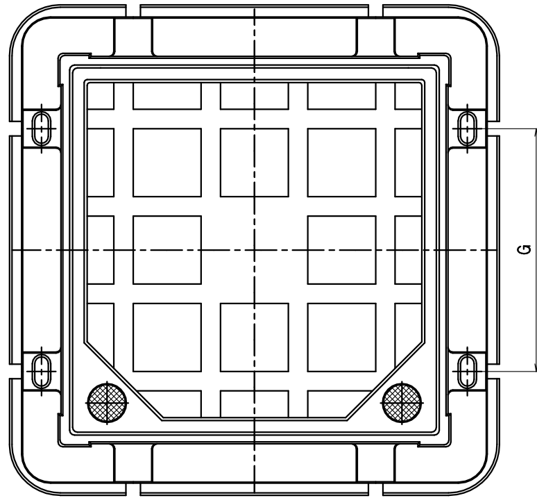
アンカー穴詳細図
