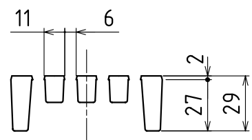
A-A矢視図
