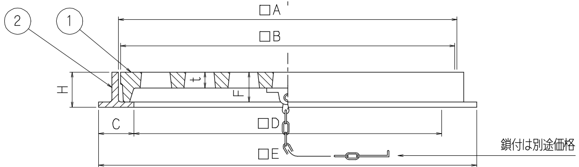
寸法表
