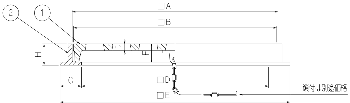
寸法表
