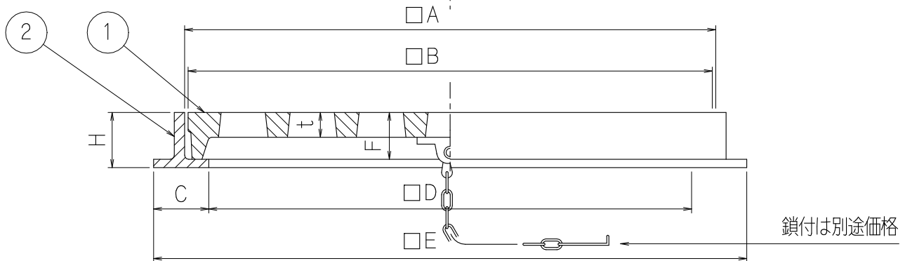
寸法表
