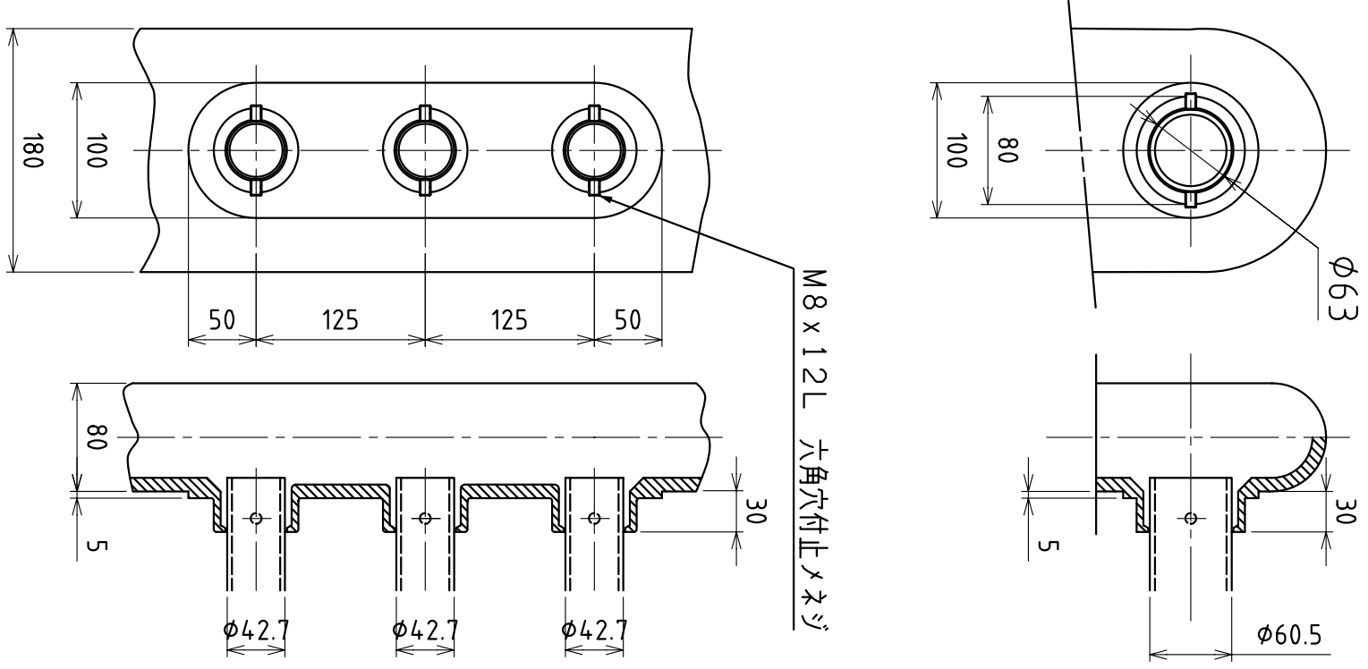
パイプ固定部 詳細図 S=1/5
