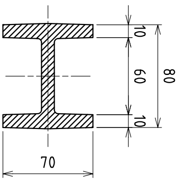
B断面図
