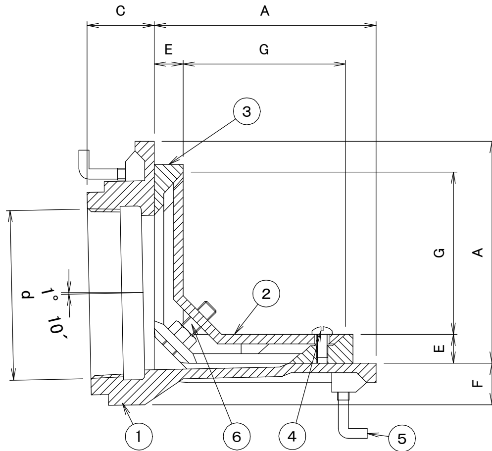
寸法表
