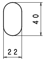
アンカー穴詳細 S=1:2
