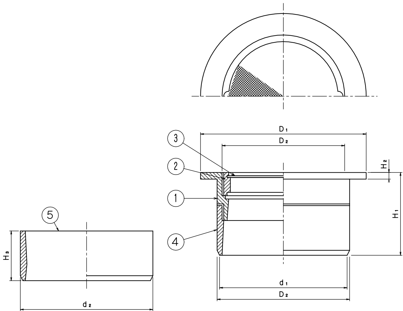
寸法表
