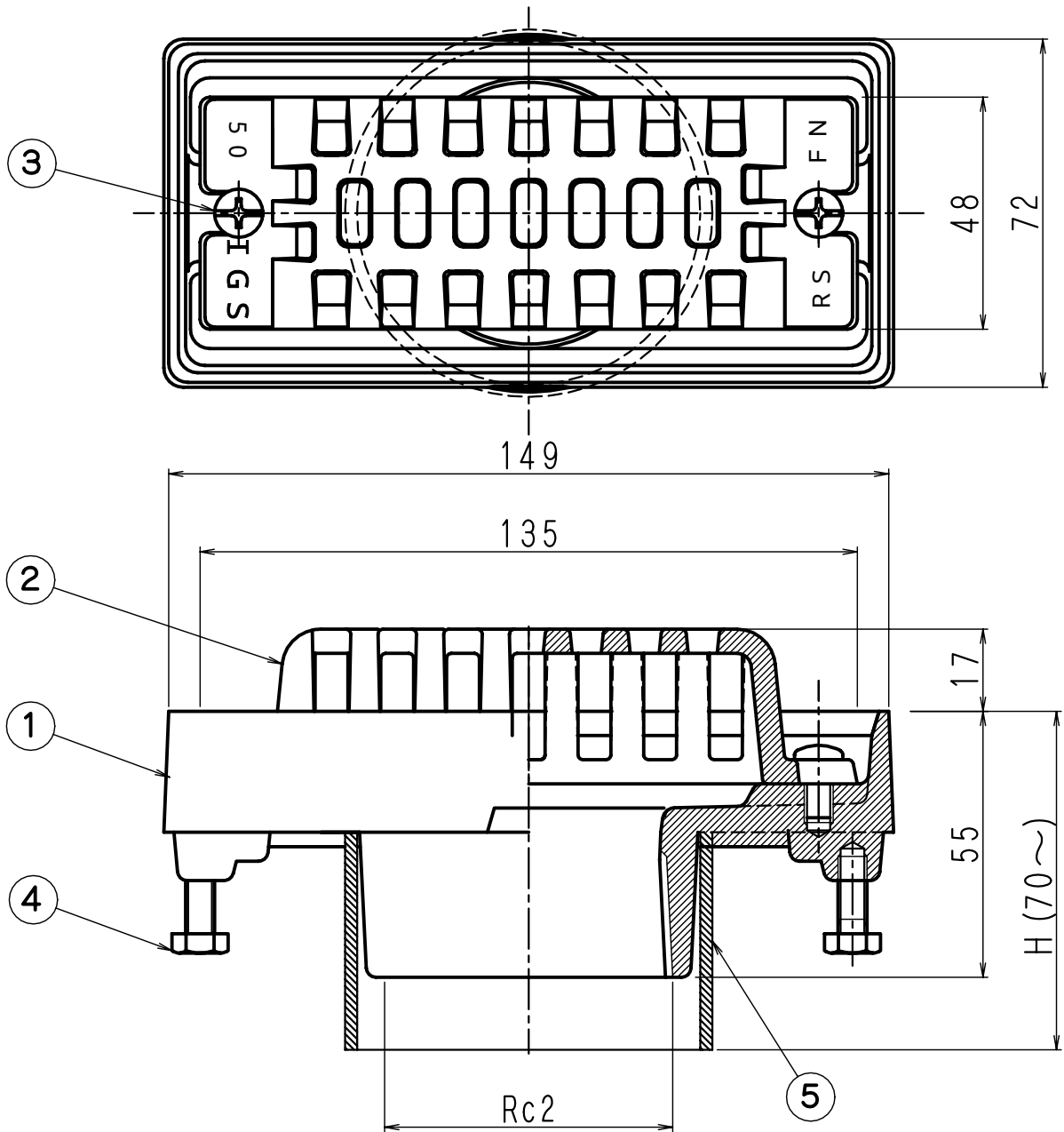
部品表
