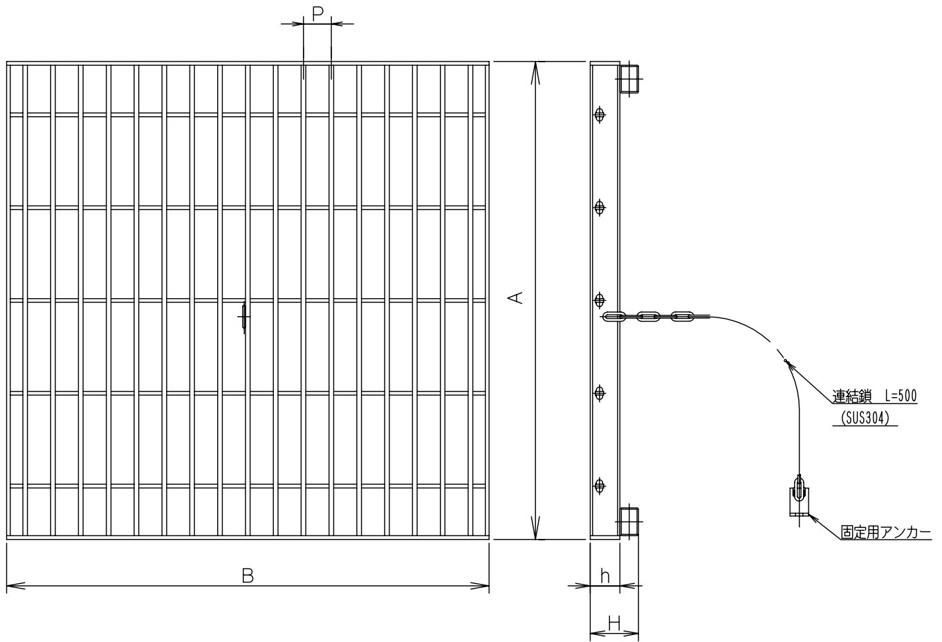
図例：SAGCD 45-2 P30 T2荷重
