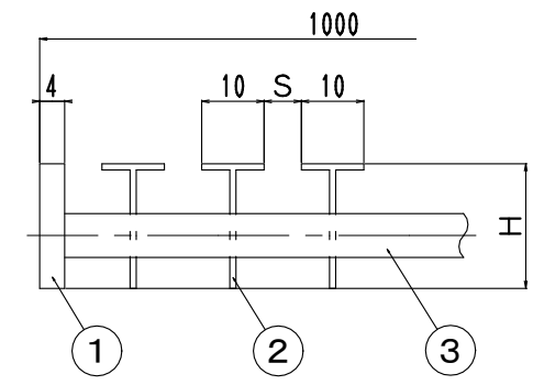
断面図
