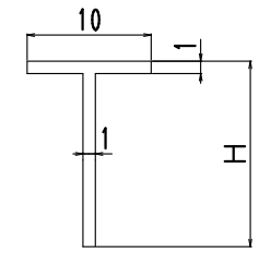
メインバー断面詳細図
