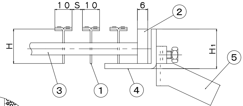
断面図
