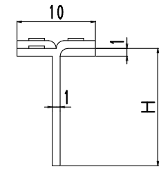
メインバー断面詳細図
