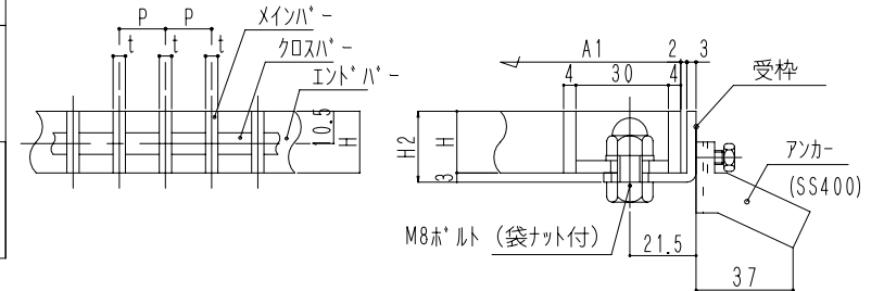
断面詳細
