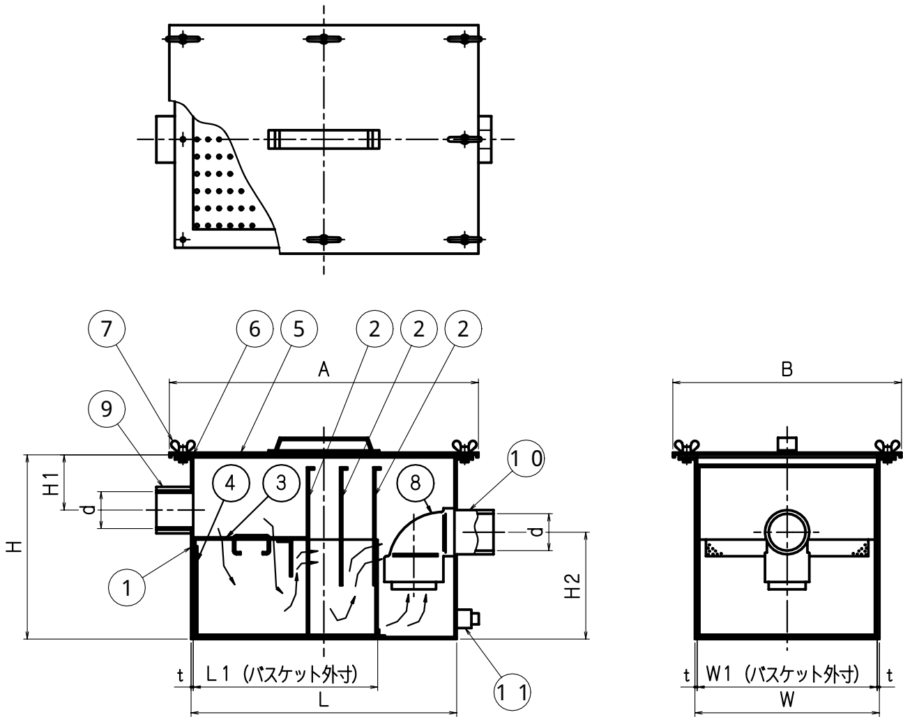
寸法表
