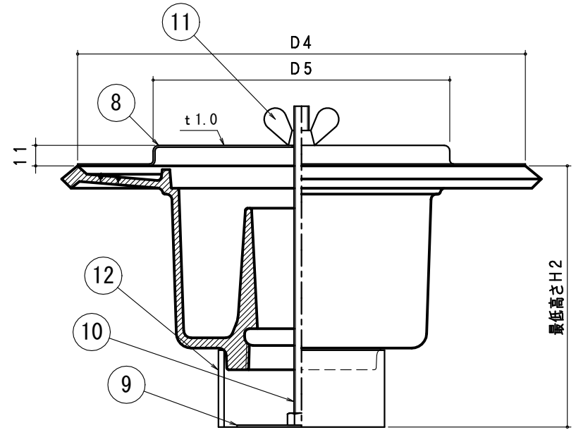
打込金具
