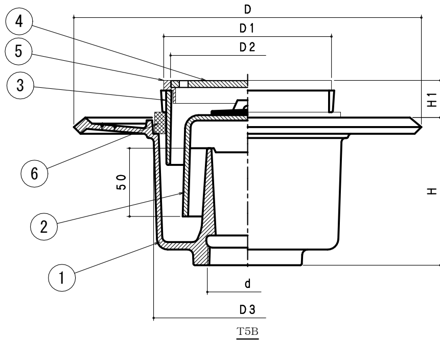
寸法表
