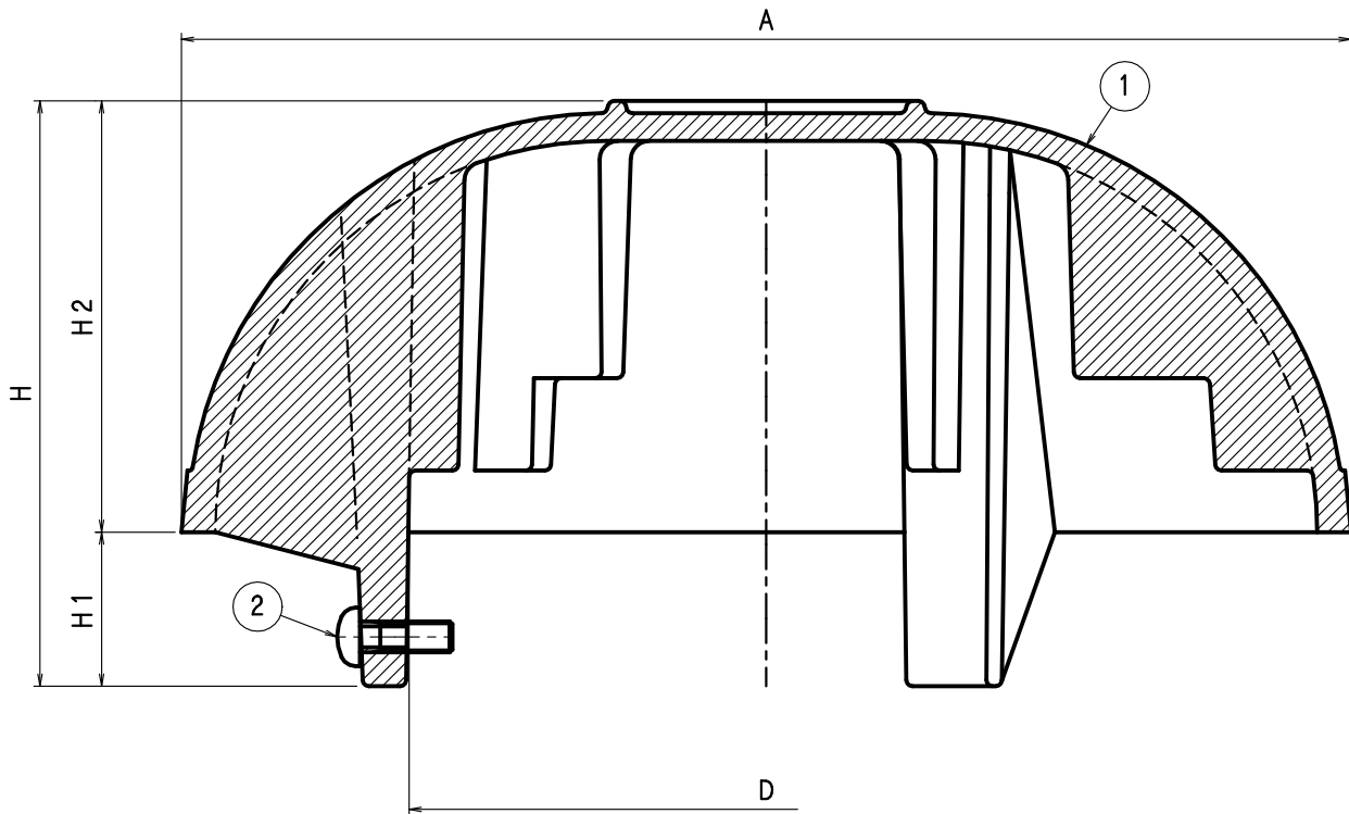
寸法表
