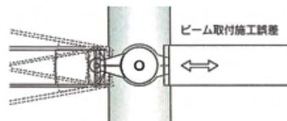
立面方向上下30° (スタンダードタイプ)
