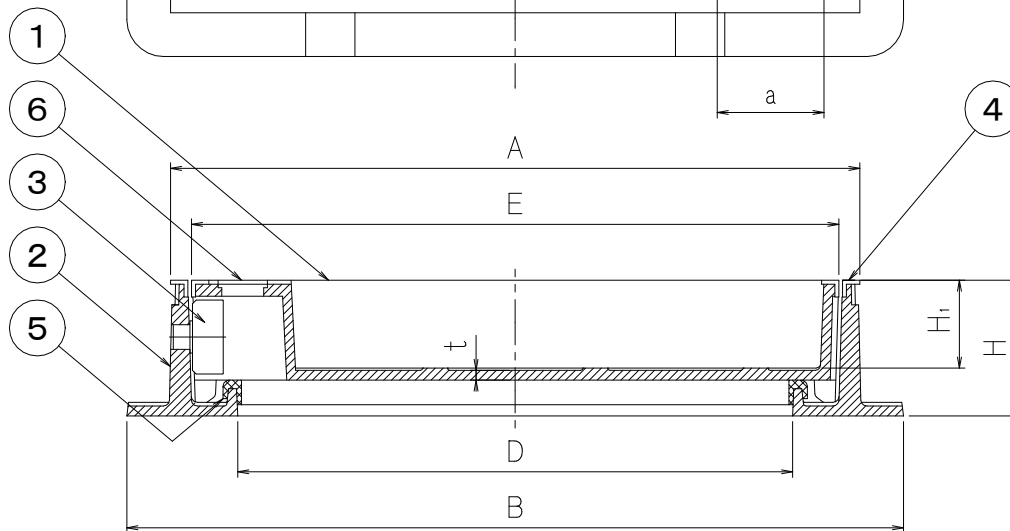
●寸法表
