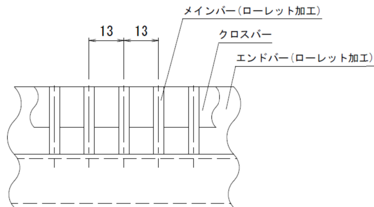
断面詳細
