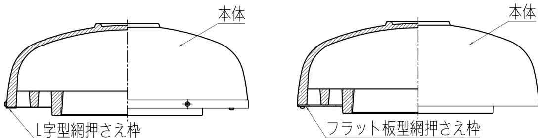
図 2 変更後品
